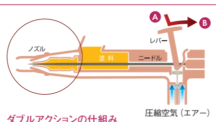
ダブルアクションの仕組み
